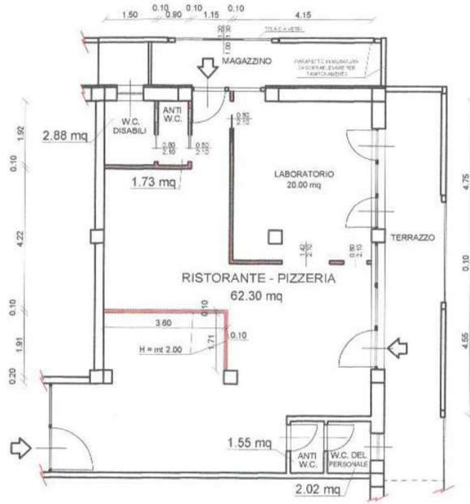
PIANTA PIANO – FUORI SCALA
