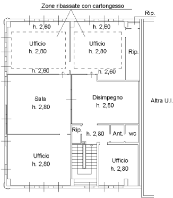
PIANO PRIMO
